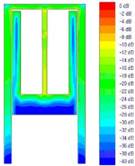
(b) 부착 대상물체 부착시의 ADDA의 전류 분포 (b) The current distribution of the ADDA on a dielectric material
