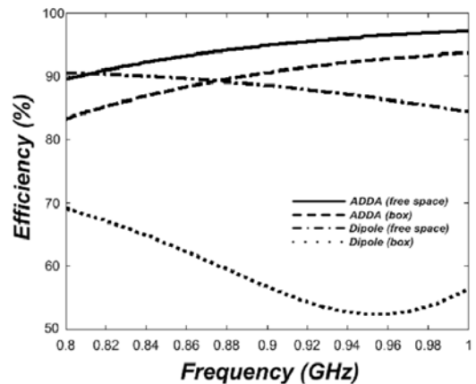
그림 4. ADDA 및 다이폴 안테나의 효율 특성 Fig. 4. The efficiency of the ADDA and the dipole tag antenna.
