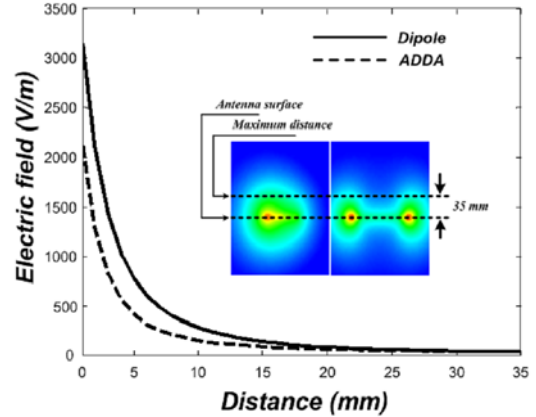
그림 6. 안테나로부터의 거리에 따른 근접 전계
