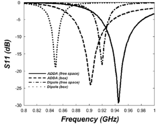
그림 3. ADDA 및 다이폴 안테나의 반사 손실 특성 Fig. 3. The return loss of the ADDA and dipole tag antenna.
