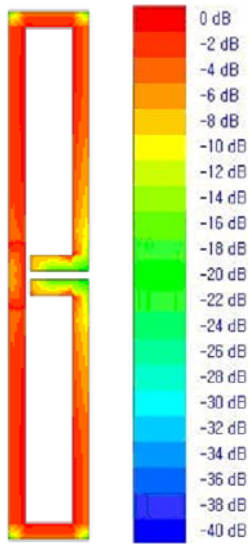
(c) 자유공간에서의 다이폴 안테나의 전류 분포 (c) The current distribution of the dipole tag antenna in free space
