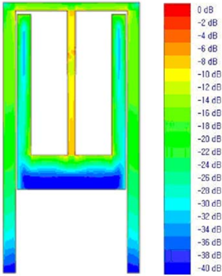
(a) 자유공간에서의 ADDA의 전류 분포 (a) The current distribution of the ADDA in free space
