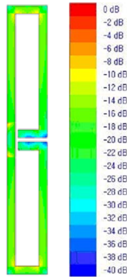
(d) 부착 대상물체 부착시의 다이폴 안테나의 전류 분포 (d) The current distribution of the dipole tag antenna on a dielectric material
